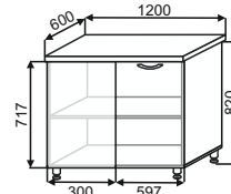
ШНУ 1200 1200x850x600
