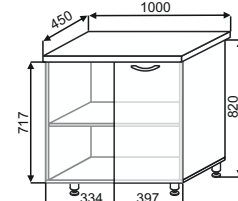
СМГУ 1000 1000x850x450
