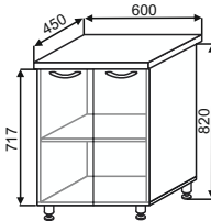
СМГ 600 600x850x450
