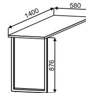
БС 1400 580x876x1400
