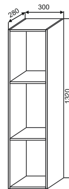
ШВО 300 300x1320x280
