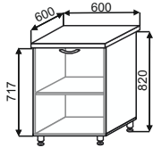
ШН 601 600x850x600
