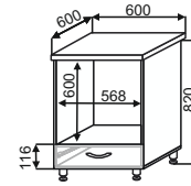
ШНД 600 600x850x600
