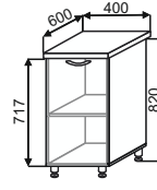
ШН 400 400x850x600
