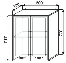
ШВС 800 800x720x300
