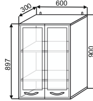
ШВС(2) 600 600x900x300
