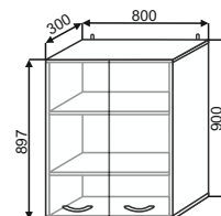
ШВ(2) 800 800x900x300
