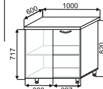
ШНУ 1000 1000x850x600
