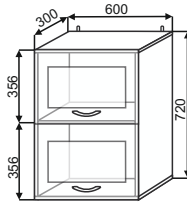
ШВБС 600 600x720x300
