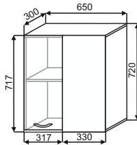
ПУГ 650 650x720x300
