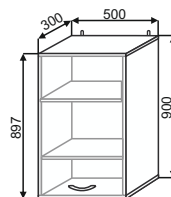
ШВ(2) 500 500x900x300
