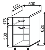
ШН(1)Я 500 500x850x600
