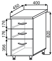
СМГЯШ 400 400x850x450
