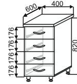
ШНЯ(4) 400 400x850x600
