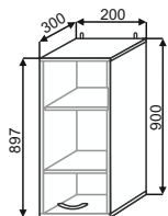
ШВ(2) 200 200x900x300
