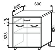
ШН(1)Я 600 600x850x600
