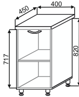
СМГ 400 400x850x450
