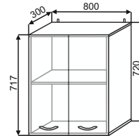
ШВ 800 800x720x300
