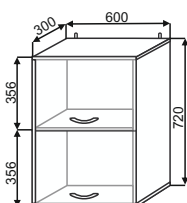
ШВБ 600 600x720x300
