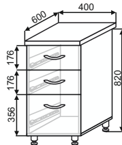
МНЯ(3) 400 400x850x600
