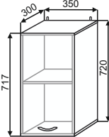
ШВ 350 350x720x300
