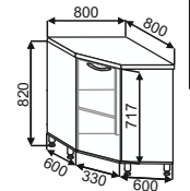
ШНУ 800x800 800x850x800
