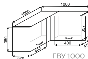
ГВУ 1000 1000x360x570
