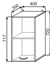
ШВ 400 400x720x300
