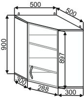
ШВУ(2) 500x500 500x900x500
