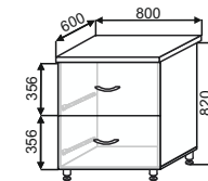
ШН2К 800 800x850x600
