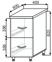
МН2К 400 400x850x600
