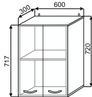
ШВ 600 600x720x300
