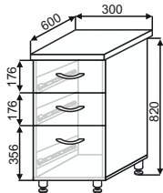
МНЯ(3) 300 300x850x600
