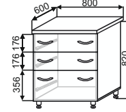
ШНЯ(3) 800 800x850x600
