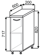
ШН 200 200x850x600
