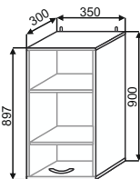
ШВ(2) 350 350x900x300
