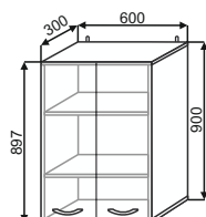
ШВ(2) 600 600x900x300
