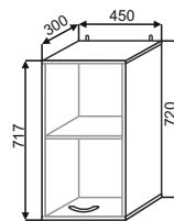
ШВ 450 450x720x300
