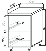
МН2К 500 500x850x600
