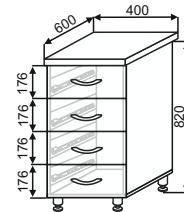
МНЯ(4) 400 400x850x600
