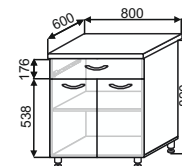
ШН(1)Я 800 800x850x600
