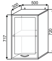
ШВС 500 500x720x300
