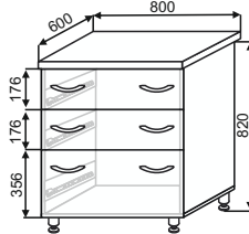
МНЯ(3) 800 800x850x600
