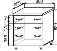
ШНЯ(3) 600 600x850x600
