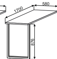
БС 1700 580x876x1700
