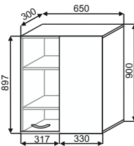
ПУГ(2) 650 650x900x300
