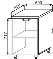
СМГ 601 600x850x450
