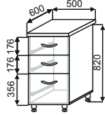
ШНЯ(3) 500 500x850x600
