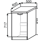
ПМ 500 500x850x600
