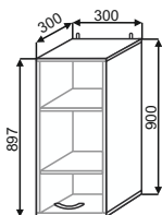
ШВ(2) 300 300x900x300
