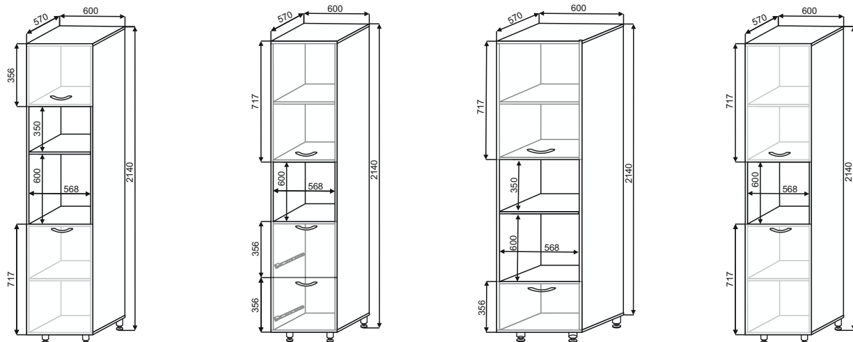
ПДШМ 600 600x2140x570
