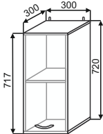
ШВ 300 300x720x300
