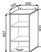
ШВ(2) 450 450x900x300
