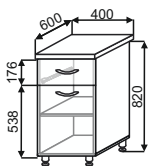
ШН(1)Я 400 400x850x600
