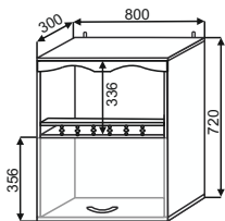
ШВПД 800 800x720x300
