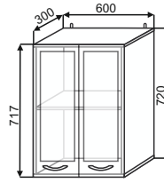
ШВС 600 600x720x300
