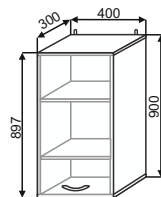
ШВ(2) 400 400x900x300
